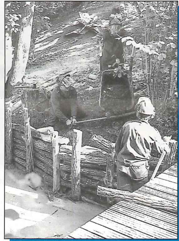
Renforcement des berges sous le Terrain d'Aventures.
