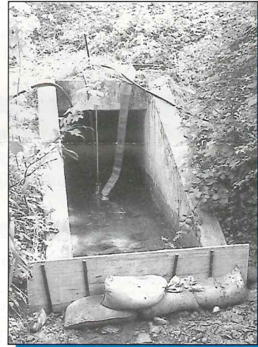
Assèchement du lit de la rivière pendant les travaux.
